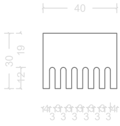
PIANTA
